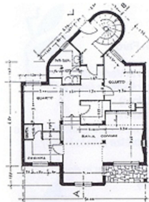
Grundriss Erdgeschoss
